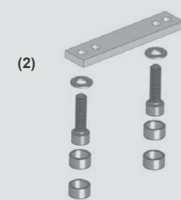
Horizontal: usar regleta para capitel reforzado Orizzontale: usare piastrina per capitello rinforzato
