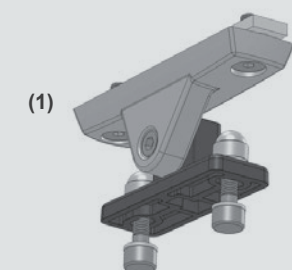
Inclinada: usar Kit anclaje articulado Inclinata: usare Kit ancoraggio articolato
